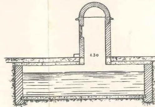
SEZIONE TRASVERSALE A-B
