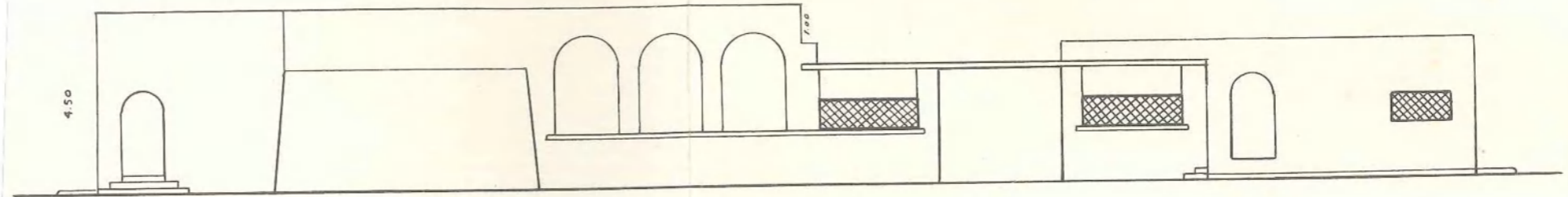
PROSPETTO
