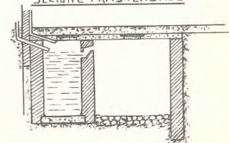
SEZIONE TRASVERSALE
