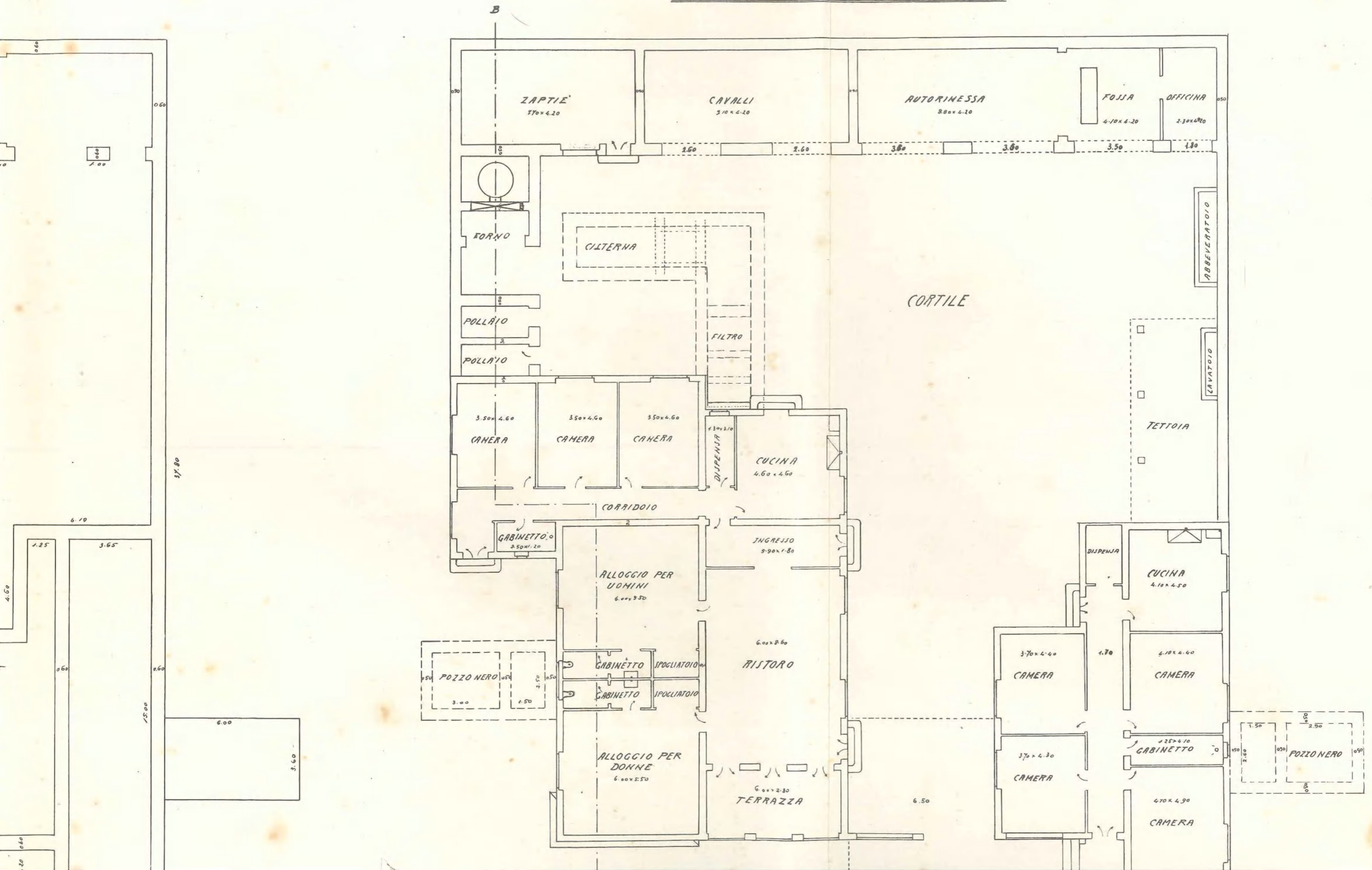
PIANTA A PIANO DELLO SPICCATO
