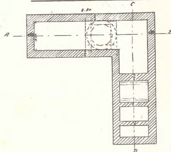
PIANTA DELLA CISTERNA
